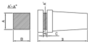
コードブッシュ寸法図 Cord Bush Dimension table
